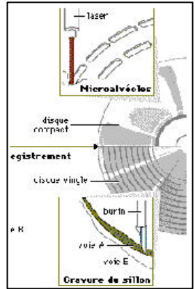
Schéma de la technique de gravage de disque
